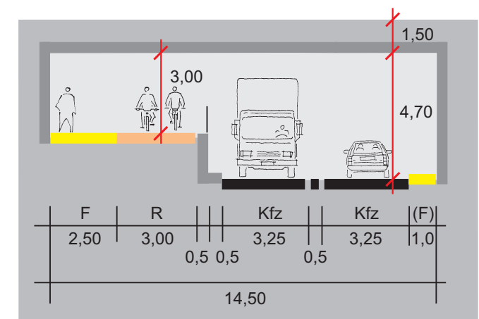
Prinzipquerschnitt Unterführung
